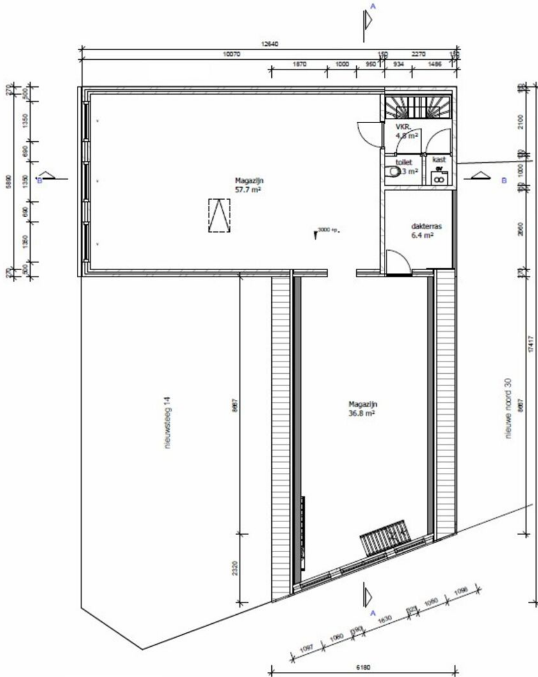
1e verdieping
