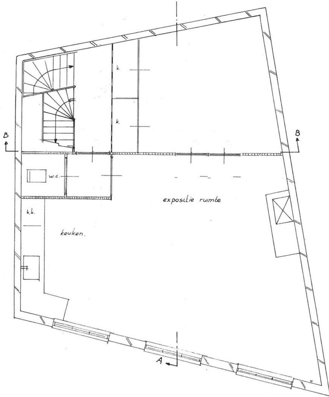
Eerste verdieping
